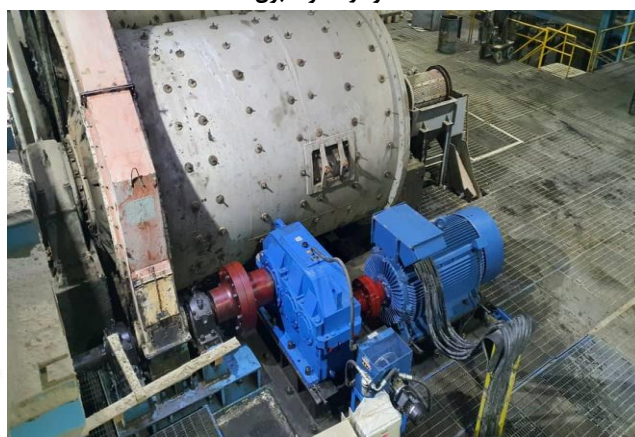
اصلاح فونداسیون و ساخت کویلینگهای جدید برای آسیا گلوله ای
