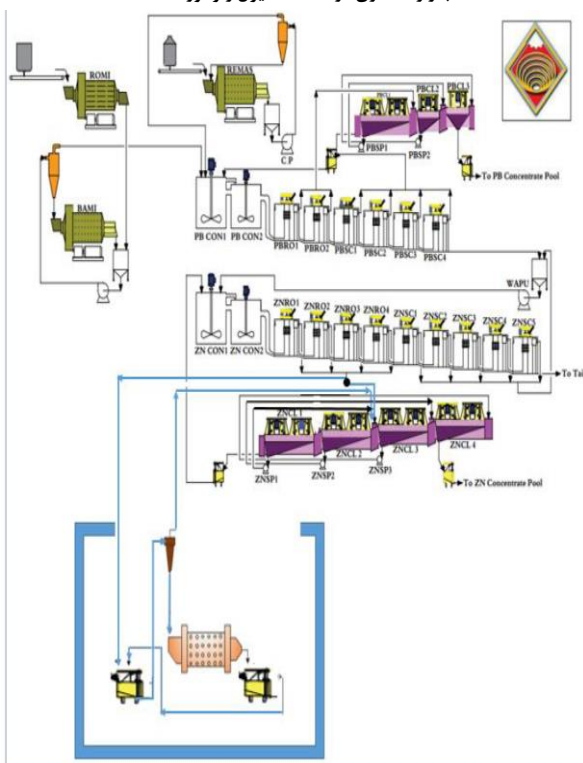
مدار ریگراند در کارخانه ۲
